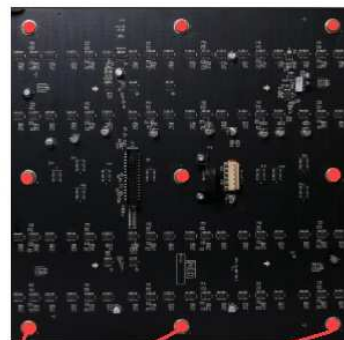
Afficheur vue arrière
